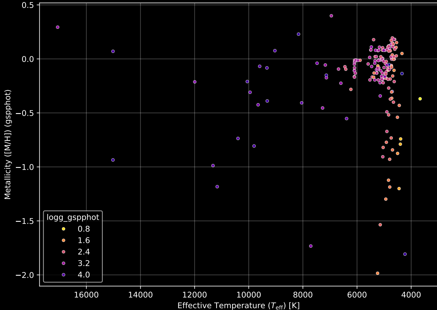
APOGEE DR17 Field: [116-04] Stellar Population Parameters (n= 173)
